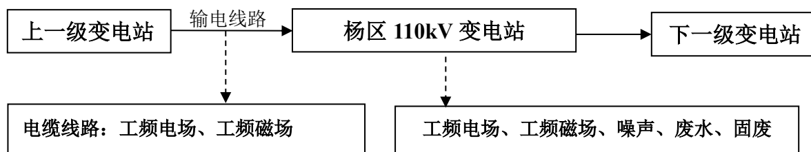
图 1 常州杨区 110kV 变电站#2 主变扩建输变电工程工艺流程及产污环节示意图
