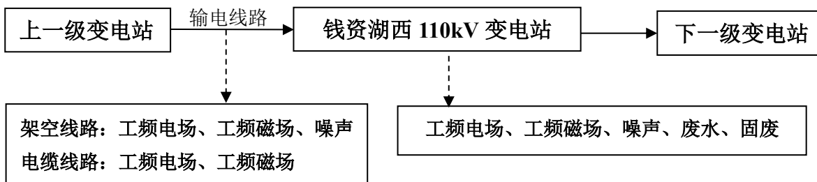
图 1 常州钱资湖西 110kV 输变电工程工艺流程及产污环节示意图
