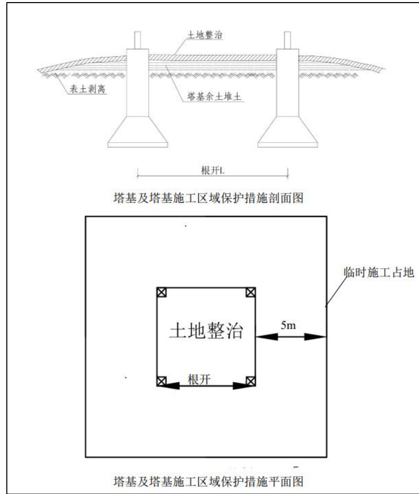
附图 10 本项目环境保护设施、措施布置图（塔基及塔基施工区域）
