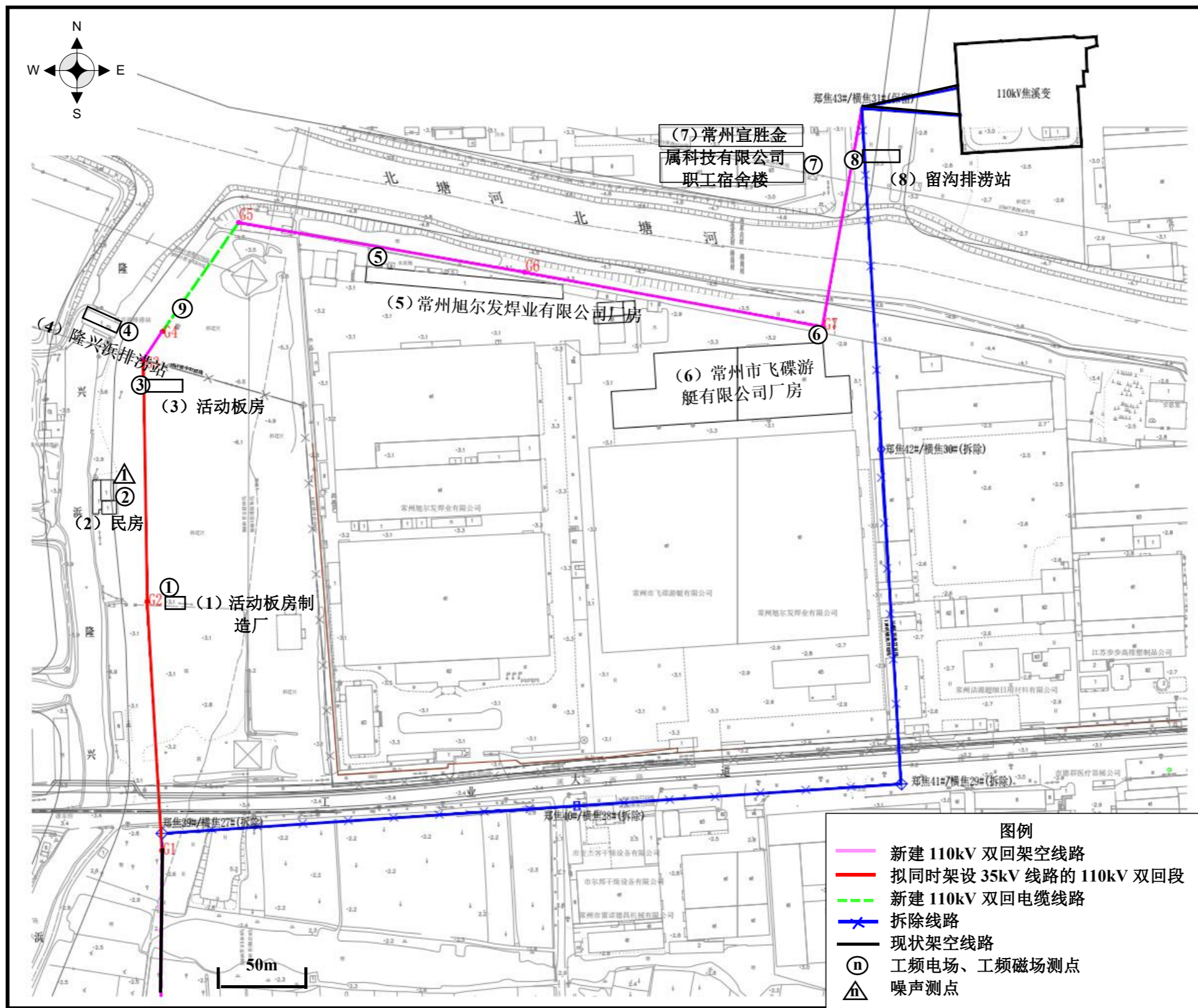
附图 3 本项目线路路径图及工频电场、工频磁场、噪声检测点位图
