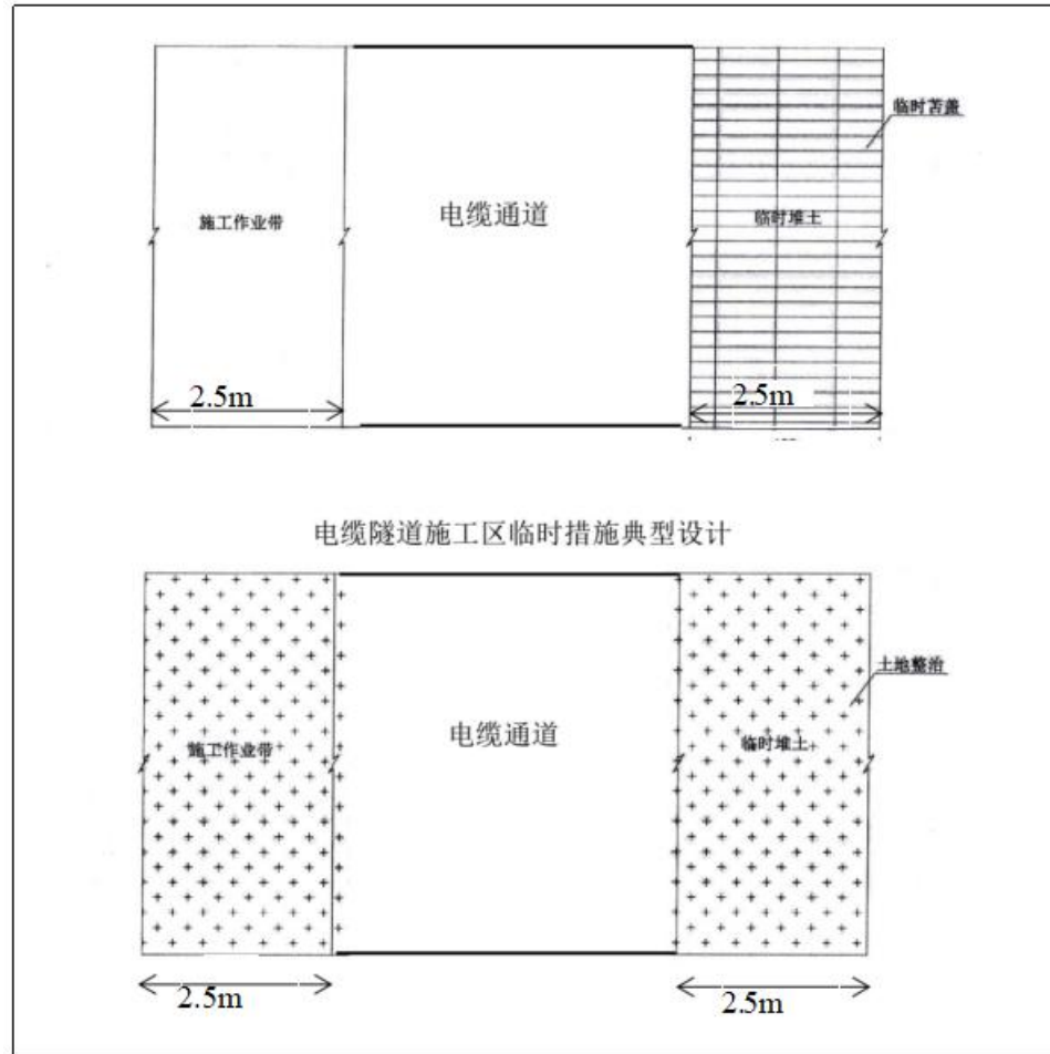
附图 11 本项目环境保护设施、措施布置图（电缆通道及施工区）
